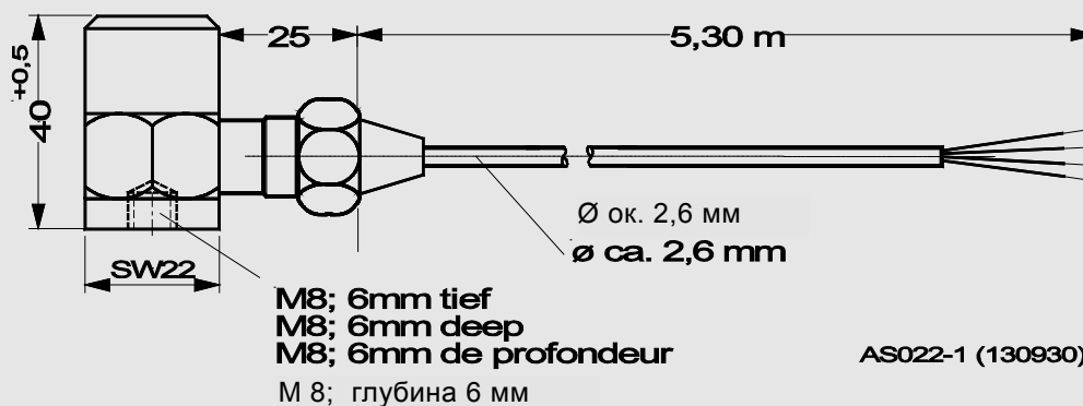
Abb. 1 Beschleunigungs-Sensor AS - 022
